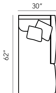
RAF CHAISE TASU50147-42-30 W 30 x D 62 x H 36 in
